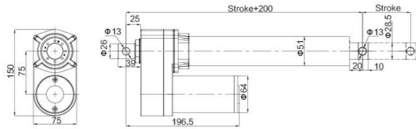
安装尺寸 | Installation Dimension
