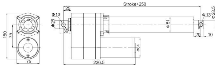
安装尺寸 | Installation Dimension
