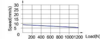
负载与速度工作图 | Load VS Speed
