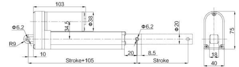
安装尺寸 | Installation Dimension
