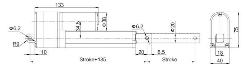
安装尺寸 | Installation Dimension
