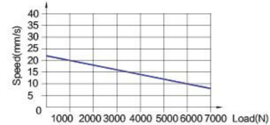
负载与速度工作图 | Load VS Speed
